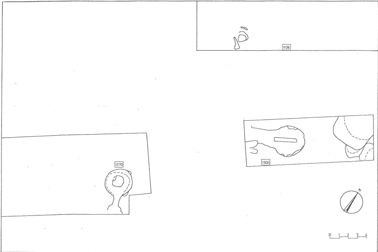
Figure 3 - Planta de los hornos que produjeron las cerámicas ibéricas (u.e. 1136, 1504) y las ánforas de tipo PE (u.e. 1270).
