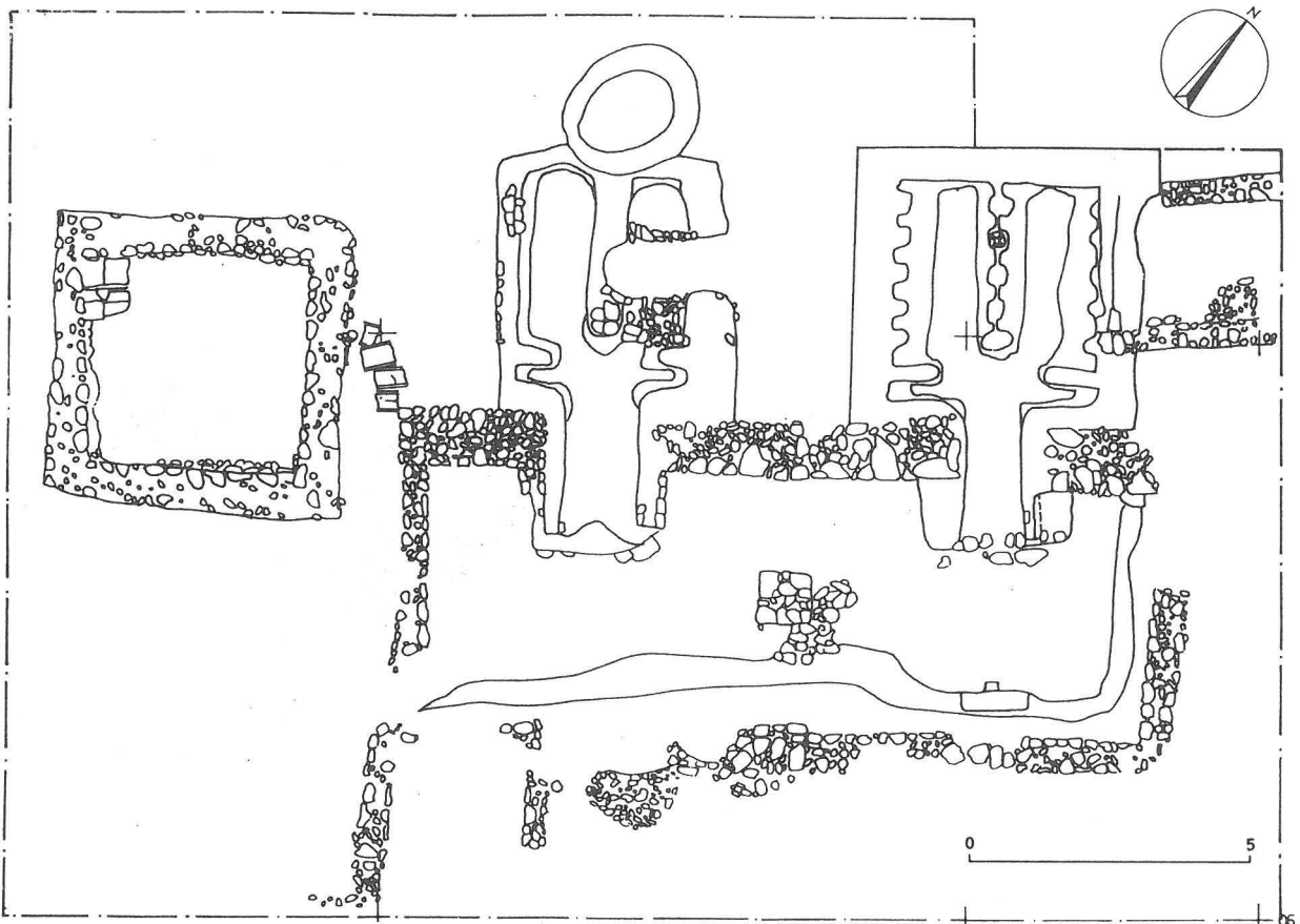
Figure 4 - Planta del taller de ánforas del siglo I.
